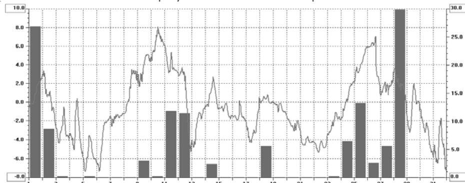
Průběh teploty a denního množství srážek v prosinci 2016
